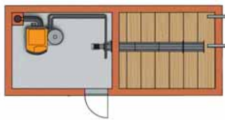
Le système d'aspiration collecte les pellets au bout de la vis d'extraction et les transporte jusqu'au réservoir journalier.
