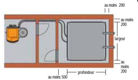
L'espace de stockage ne doit pas nécessairement se trouver directement à côté de la chambre de chauffe. Le « pont d'air » peut franchir des distances correspondant à 20 m de longueur de tube.
